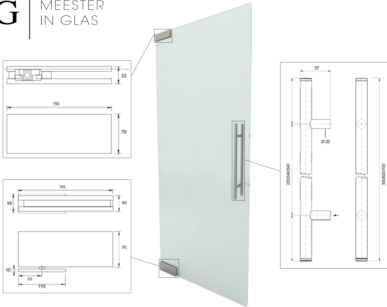
Glazen taatsdeur
